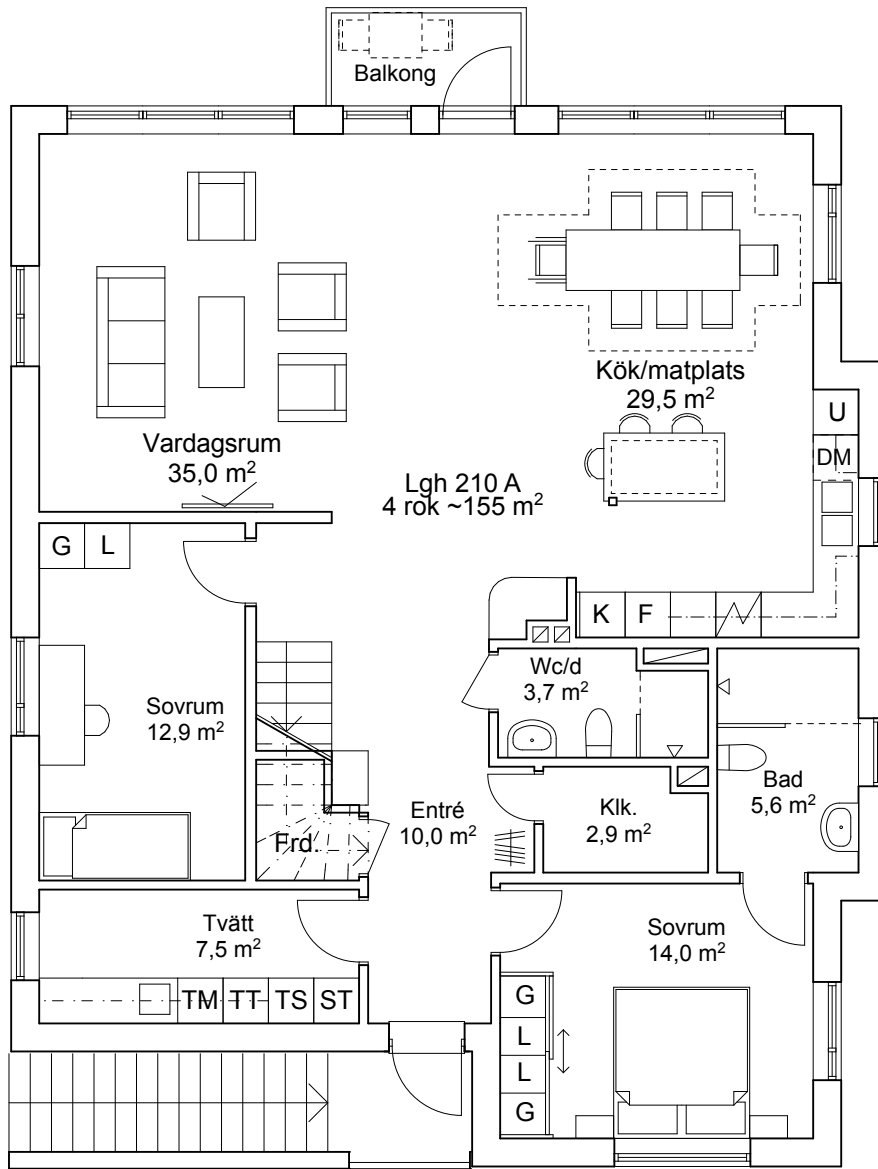
Övre plan
